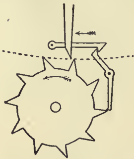
FIG. 14.—Free Escapement (old form).
